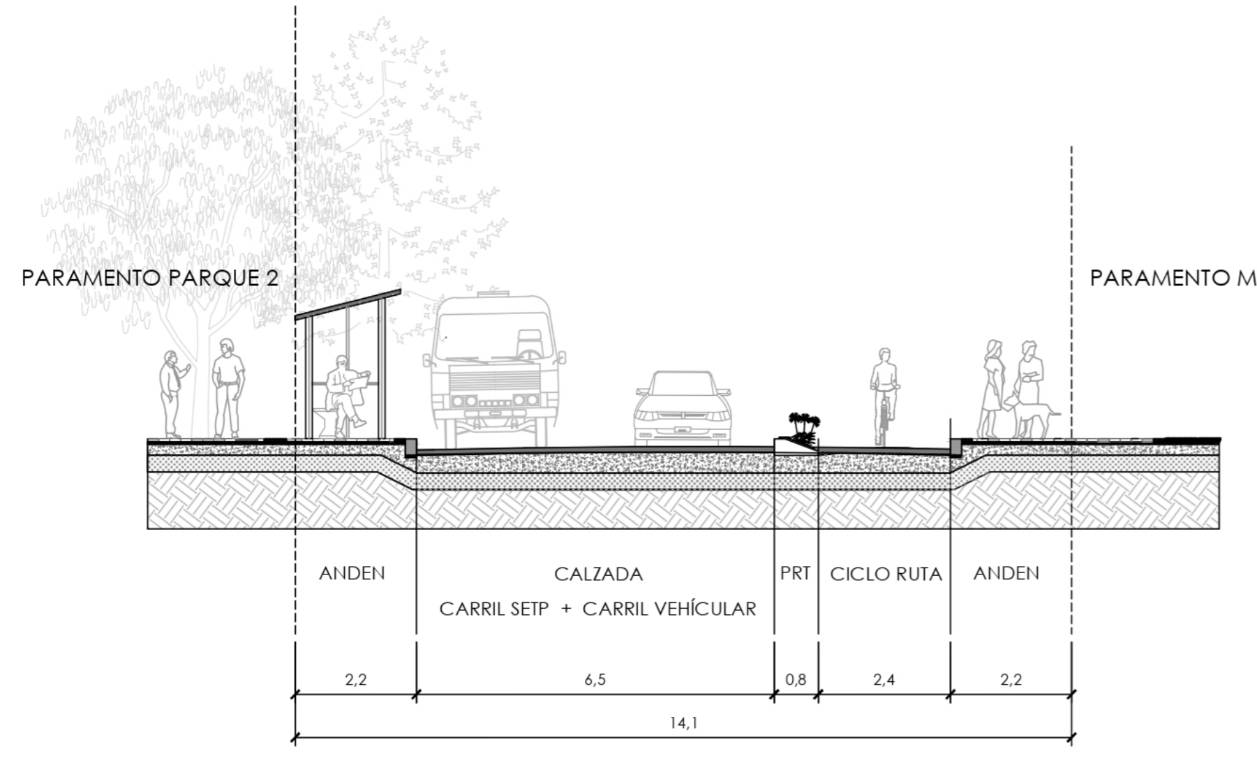
PERFIL VIAL TIPO PLAN PARCIAL LA MACARENA
